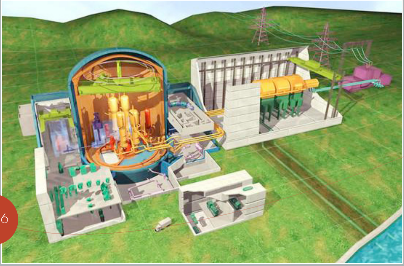
Şekil 3 VVER -1200 Nükleer Güç Santrali (yandan görünüm) (Altshuller 2006).
